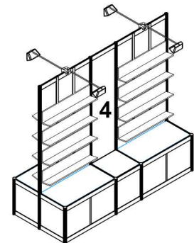
Présentoir double 2 1/2m
