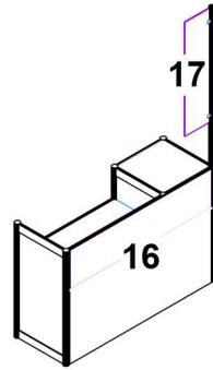
Comptoir caisse avec fanion 1 1/2m x 1/2m x 40"
